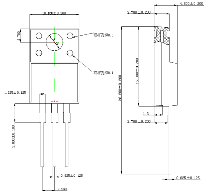
ITO-220
