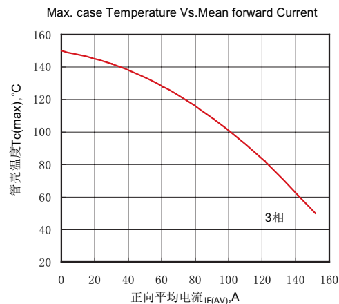
Fig.4 管壳温度与平均电流的关系曲线
