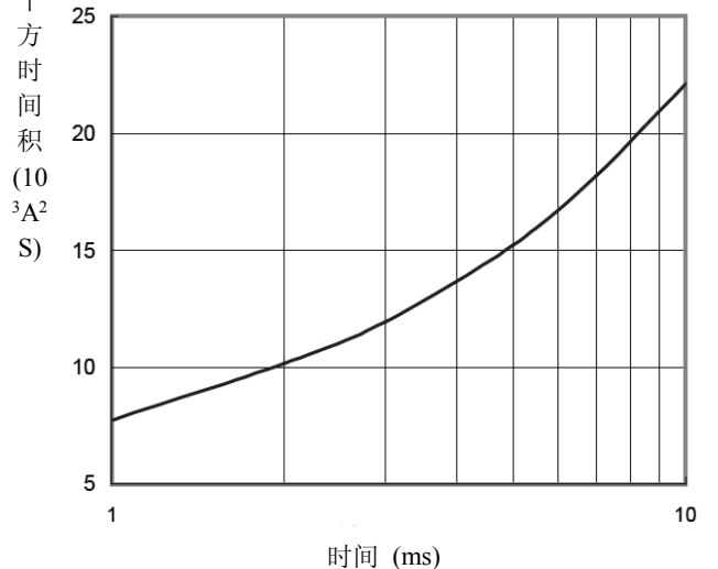
I^2t 特性曲线
