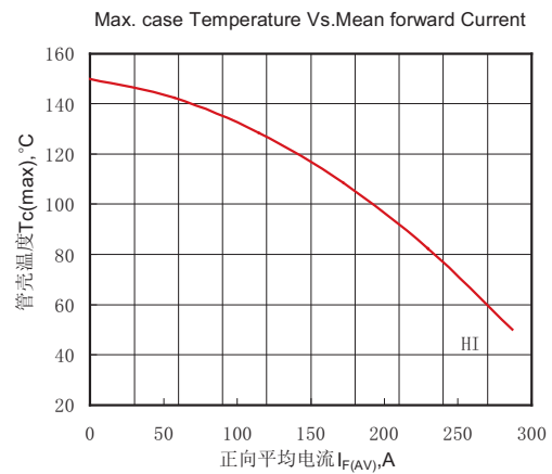
Fig.4 管壳温度与平均电流的关系曲线
